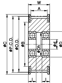
IDTS TYPE (Bearing 2 pcs.)
