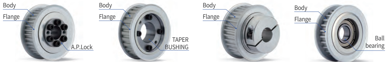
A.P.Lock Type (SPA)
