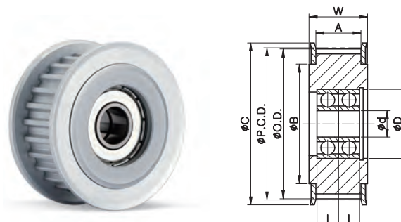
IDTC TYPE (Bearing 2 pcs.)
