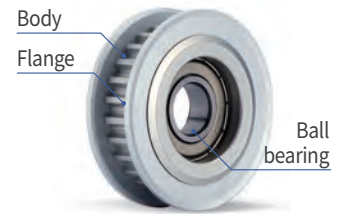
IDLER Type (ID□□)
