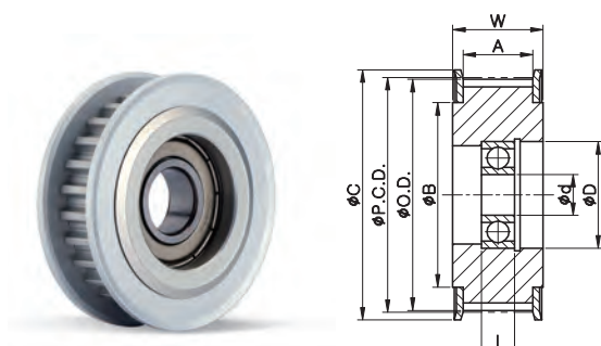
IDOC TYPE (Bearing 1 pc.)
