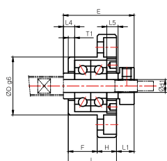
設置方法A
