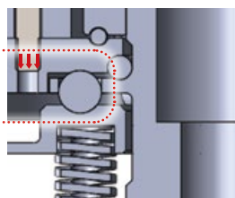
空回転駆動状態
