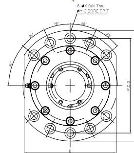
SWBK-50-G
