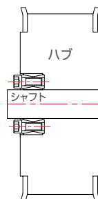
▲ SAPL-D1シリーズ装着例
