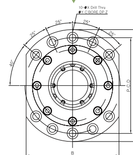
SWBK-50
