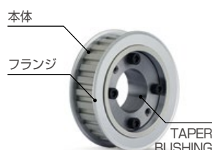
TAPER BUSHINGタイプ (SPB)
