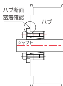
▲ SAPL-D3シリーズ装着例
