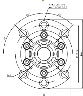
SWBK-17~SWBK30
