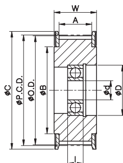
IDOC TYPE (싱글베어링)
