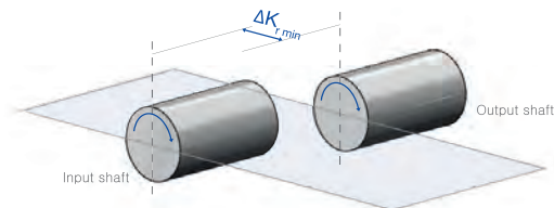
Figure 1. 슈미트 커플링의 작동을 위한 최소 편심량 확보를 위해 출력축이 평행방향으로 Offset 되어 있음
